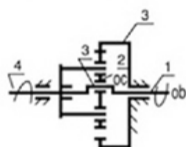
图1 传动原理 Siagram 1 Driving Principte
